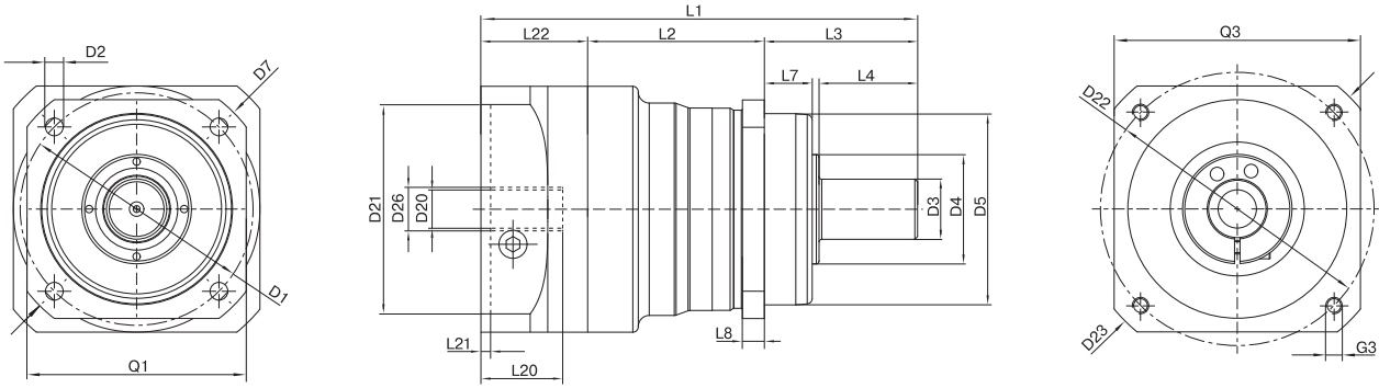
PLN090 ile aynı özelliklerde / 1-kademeli / kamasız mil / 19 mm sıkma sistemi / motor bağlantılı – 2 parçalı – dairesel üniversal flanş yapısı / B5 motor flanş tipi Drawing corresponds to a PLN090 / 1-stage / smooth output shaft / 19 mm clamping system / motor adaptation – 2-part – round universal flange / B5 flange type motor Diğer tüm çizimler www.neugart.com.tr de Tec Data Finder altında mevcuttur – All other variants can be retrieved in the Tec Data Finder at www.neugart.com
