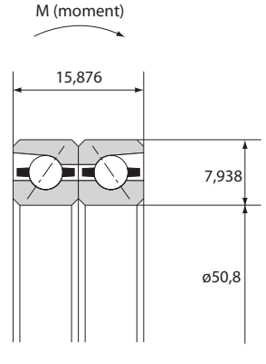
Açısallı bilyeli rulman
